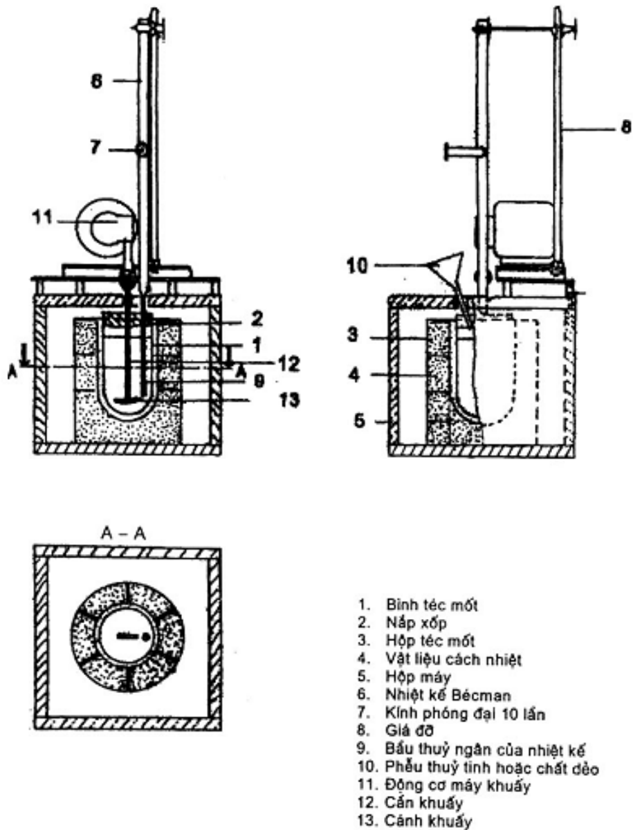
Hình 1 – Mô tả thiết bị đo nhiệt lượng
