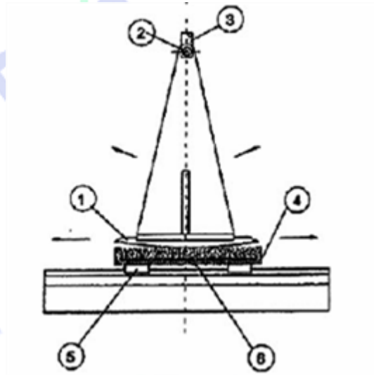
(b): Sơ đồ đầm lăn bán tự động
