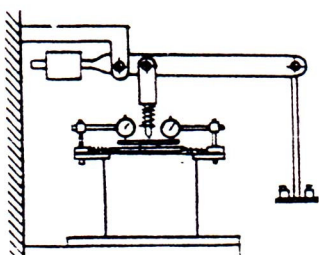
Hình B-1: Sơ đồ lắp đặt tấm ép và thiên phân kế
